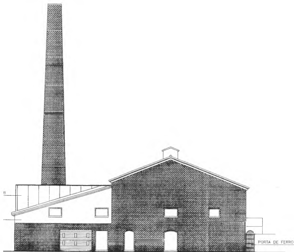
FAÇANA SUD-OEST
