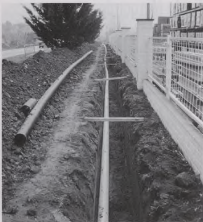
Canonada de gas de Palol d'Onyar a Quart.
